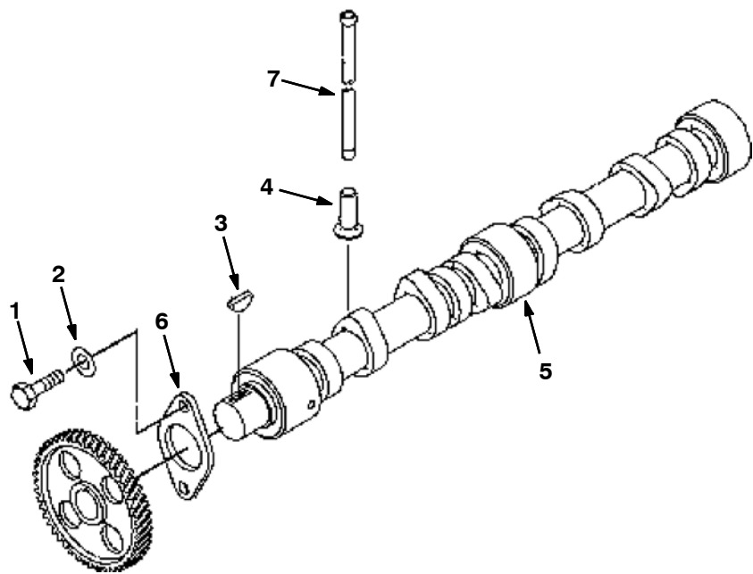
Fig. 5 - Camshaft Group
