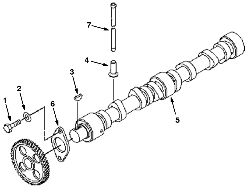
Fig. 5 - Camshaft Group
