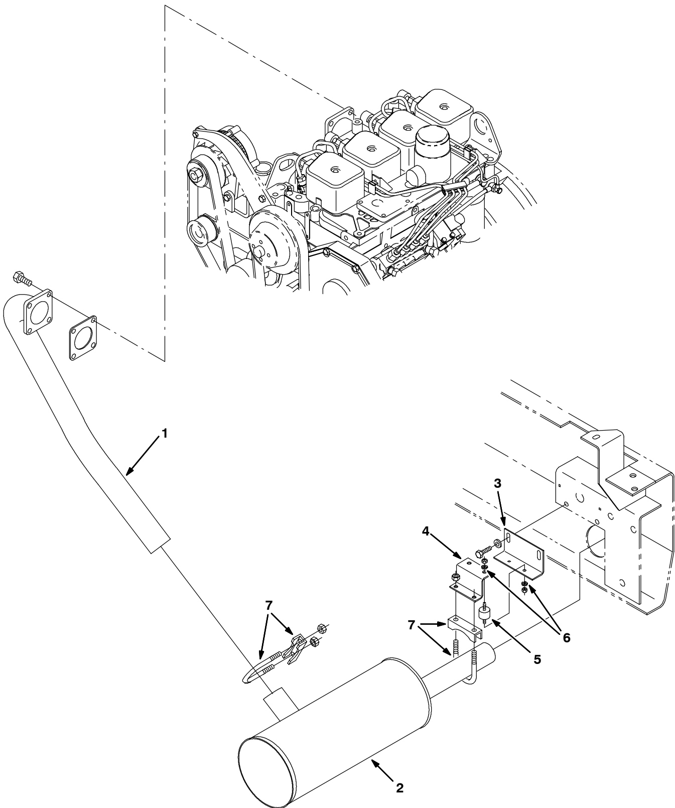
Fig. 24 - Muffler Group
