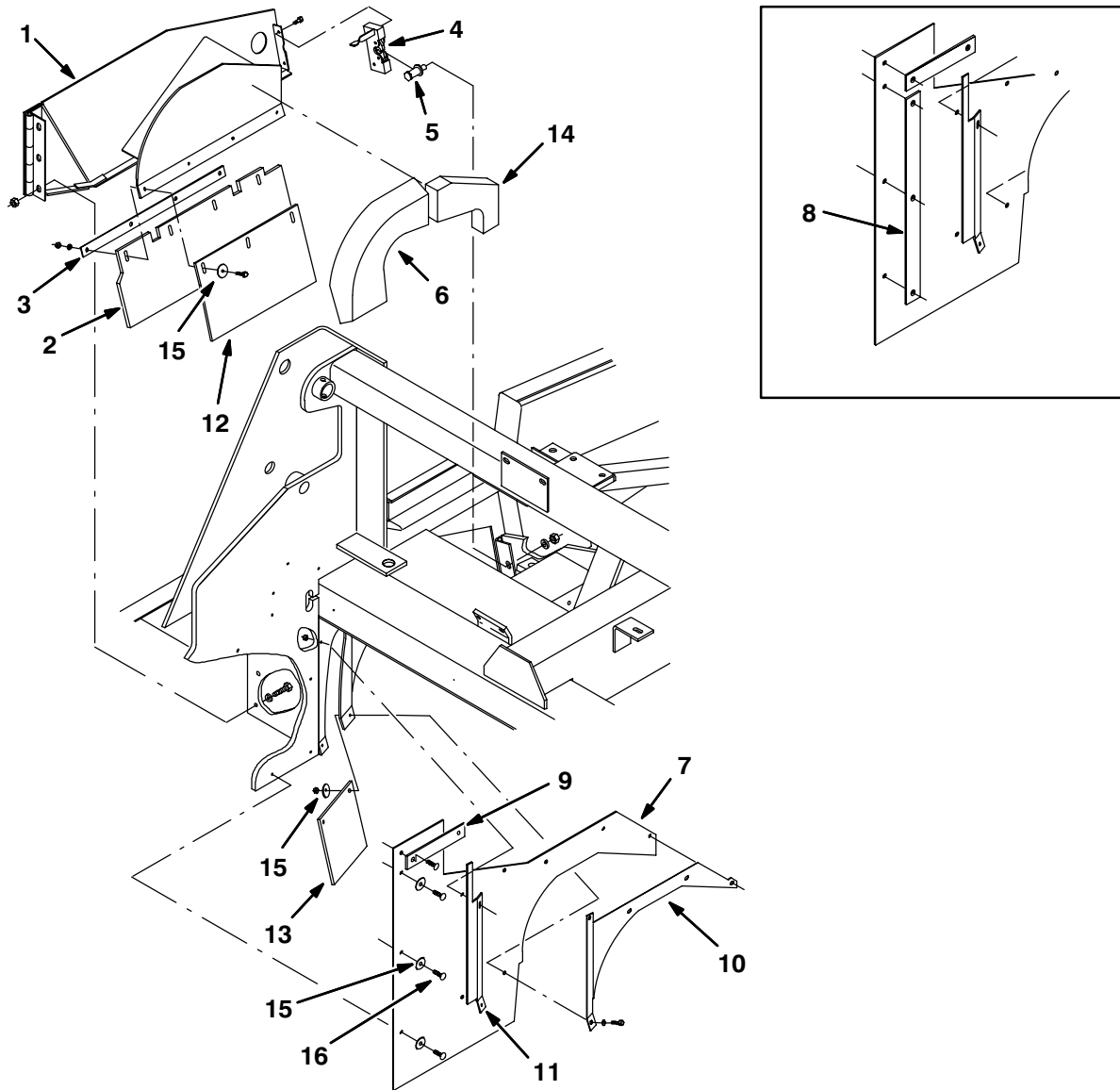
Fig. 6 – Right Brush Door Group
