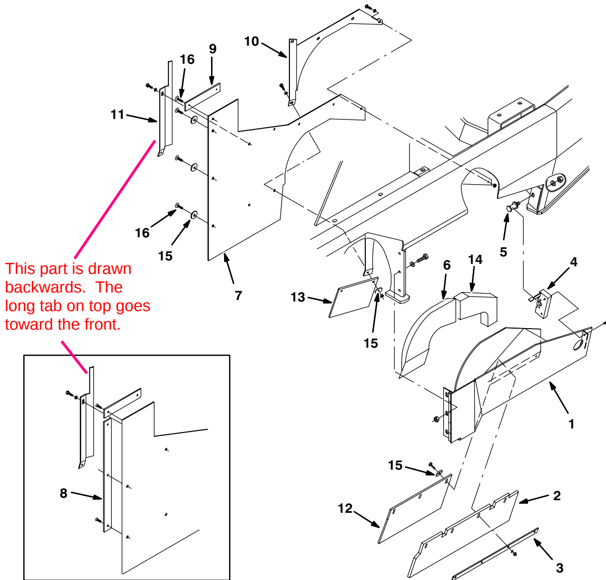
Fig. 5 – Left Brush Door Group
