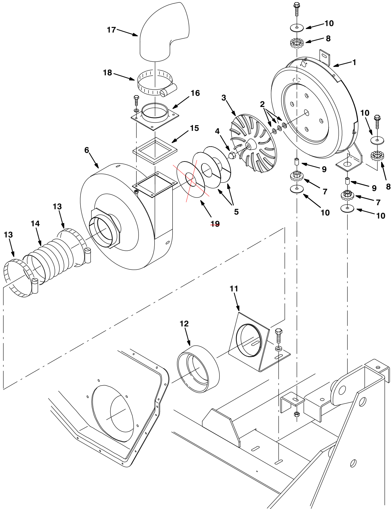
Fig. 65 – Vacuum Fan Impeller Group
